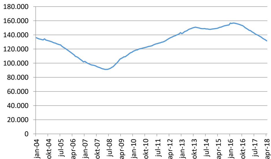
Figur 1. Antal fuldtidspersoner i kontanthjælpsystemet. Sæsonkorrigeret.
