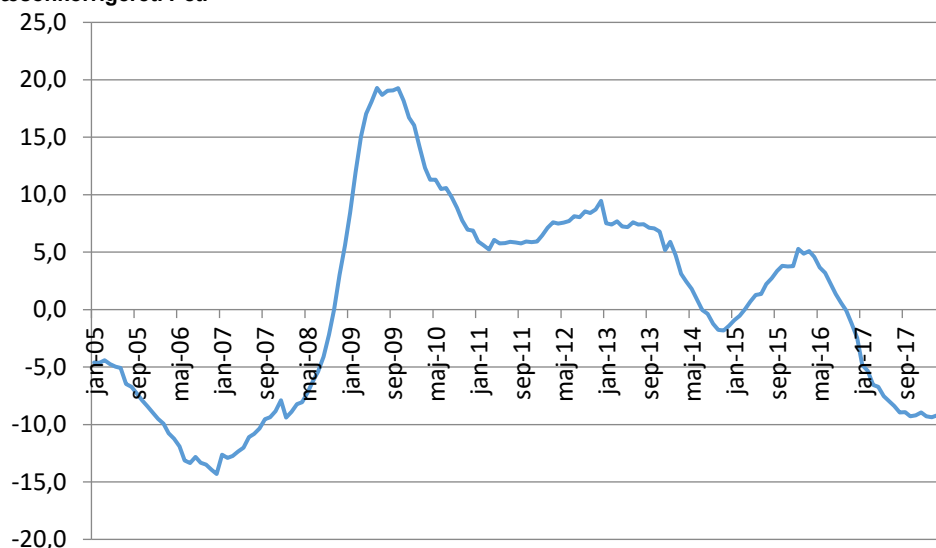
Figur 2. Årlig ændring i antal ydelsesmodtagere i kontanthjælpssystemet (fuldtidspersoner).
